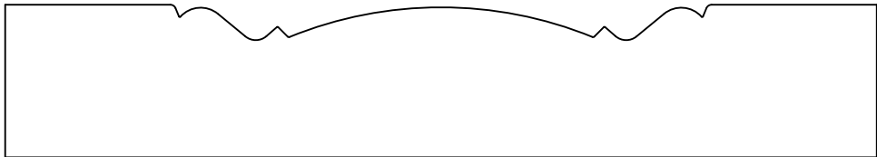
HWP1216 Rosette 0.875" x 5.000"
